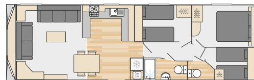
37' x 12' - 3 Bedroom
